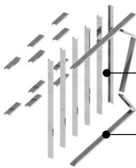
Structure du mur Profils non assemblés
